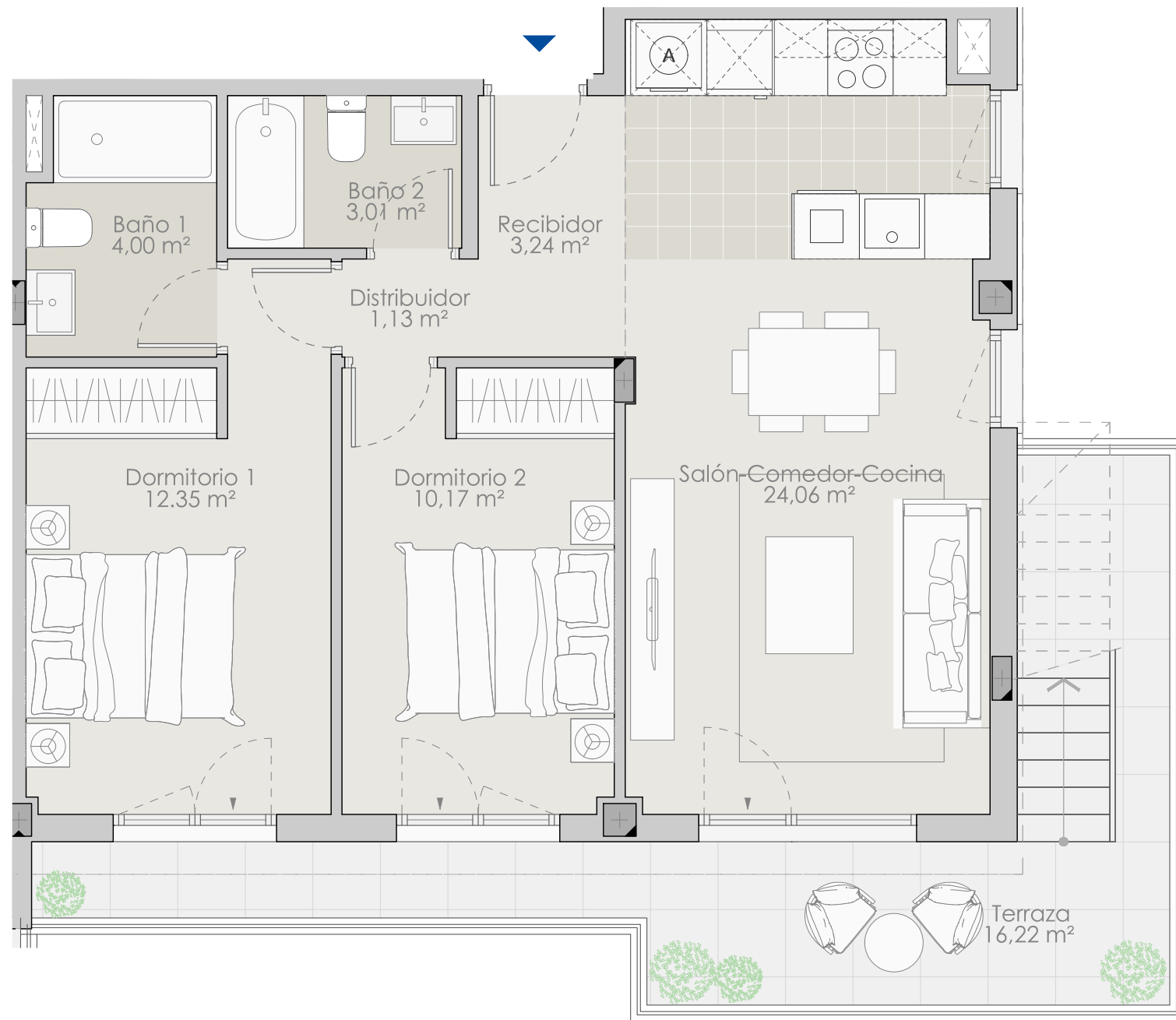
PLANTA SEGUNDA
