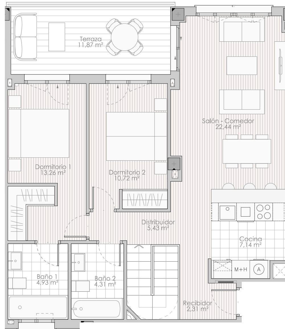
PLANTA PRIMERA
